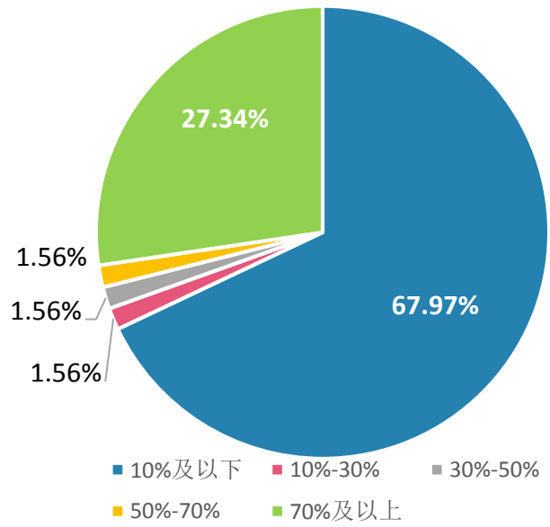
图 4.6.2. 流动比率
