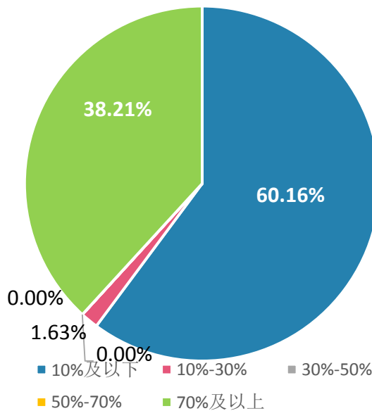
图 5.6.2 流动比率
